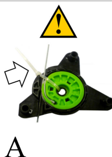
- POSIZIONE INSERIMENTO IN PORTIERA ALZACRISTALLI ELETTRICO. - POWER WINDOW INSTALLATION POSITION INTO THE DOOR.
