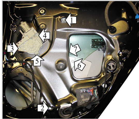
A POWER WINDOW RIGHT ALZACRISTALLI ELETTRICO DX
